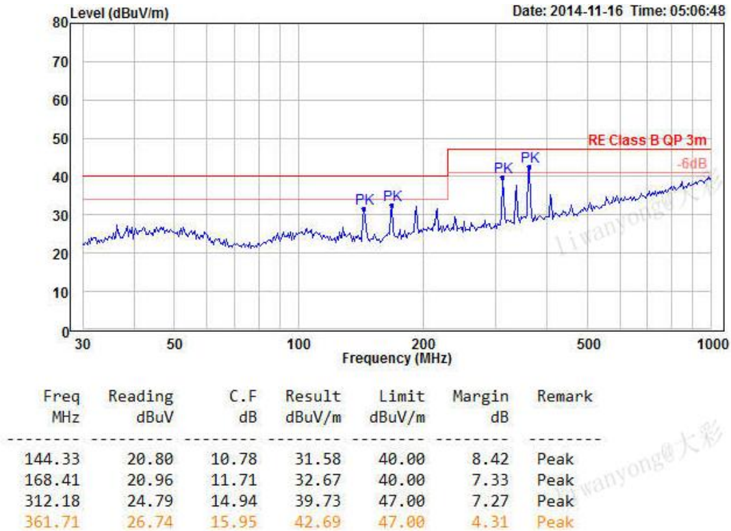
图 5-7 辐射测试垂直方向
