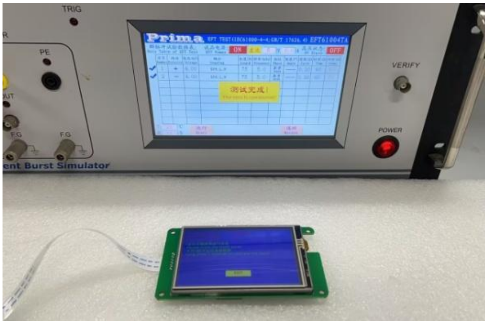
图 5-4 脉冲群测试图
