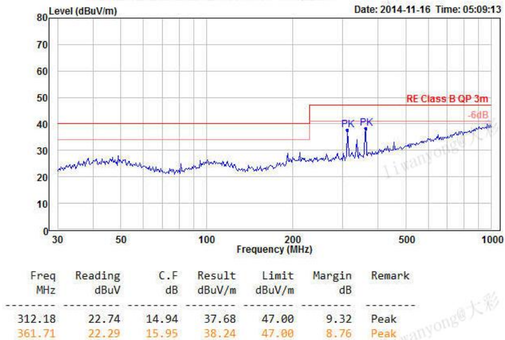
图 5-6 辐射测试水平方向
